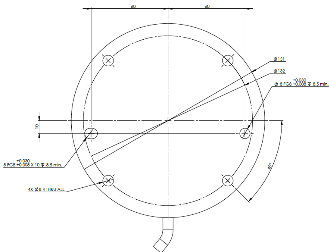
1.1: ロボットベースの底面図
